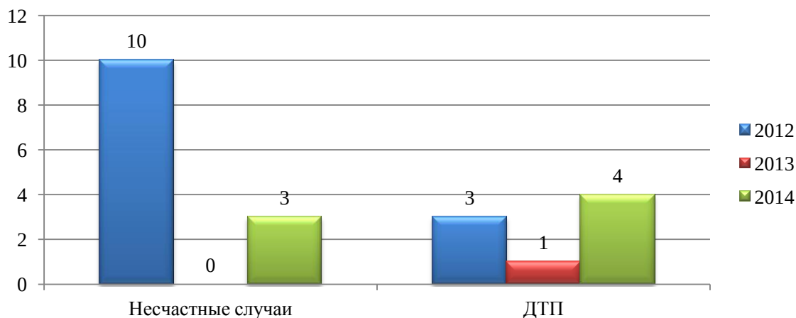
Динамика несчастных случаев, ДТП
